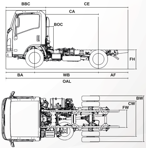
ELF 300 (RODADO DOBLE)
