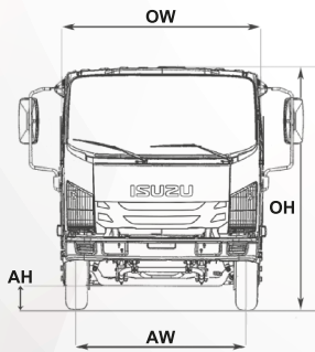
DIMENSIONES
